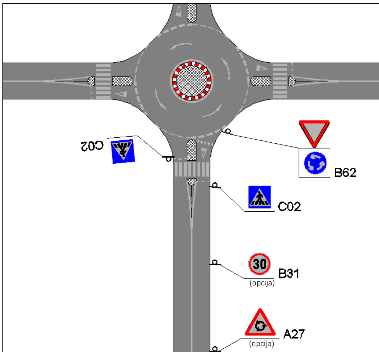
Slika F4: Primjer postavljanja prometne signalizacije na privozu mini kružnog raskrižja
