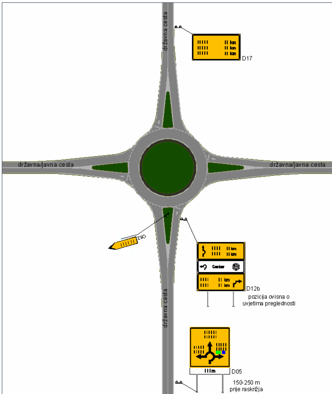
SLIKA F3: Primjer postavljanja signalizacije za vođenje prometa na raskrižju državnih cesta ili državne i javne ceste (županijske, lokalne). Znakovi upozorenja i izričitih naredbi prikazani su u prilogu F.1. i F.2.
